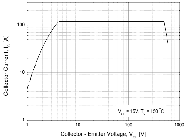
Fig. 15 RBSOA
